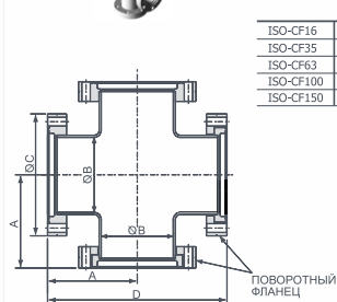
Крест ISO-CF равнопроходный поворотный Исполнение: из нержавеющей стали
