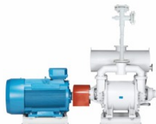
ABB-50 / ABB-50H ВОДОКОЛЬЦЕВОЙ ВАКУУМНЫЙ АГРЕГАТ
