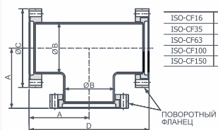
Тройник ISO-CF равнопроходный поворотный Исполнение: из нержавеющей стали
