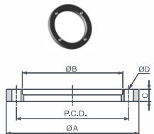
Фланец ISO-F поворотный
