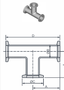
Тройник ISO-KF равнопроходный
