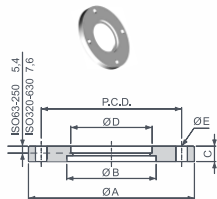
Фланец ISO-F
