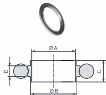
Центрирующее кольцо ISO-F в сборе
