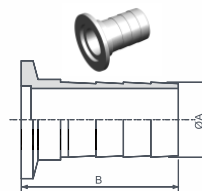
Штуцер ISO-KF с наконечником
