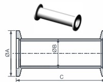
Патрубок ISO-KF
